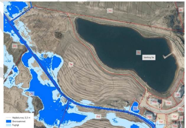
Oversvømmelse fra vandløb - sommerskybrud, 1288 l/s
